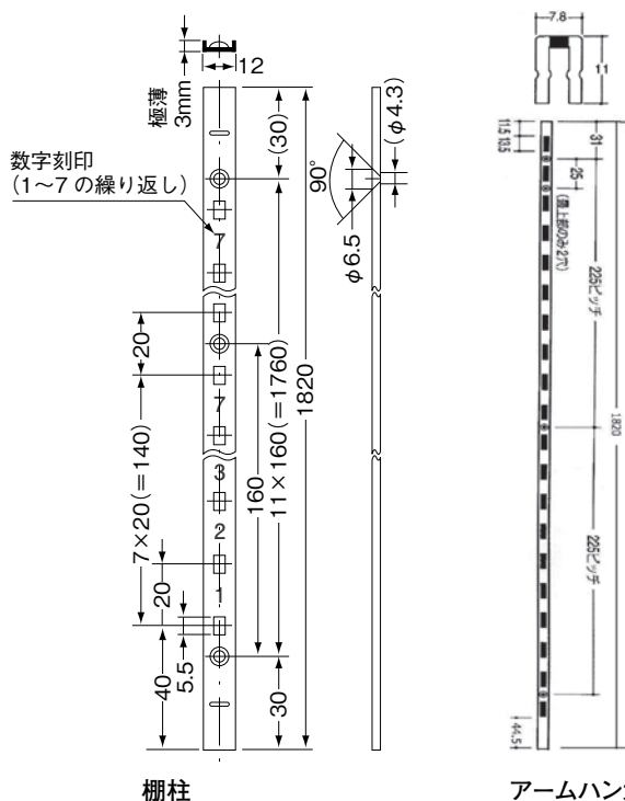
棚柱
