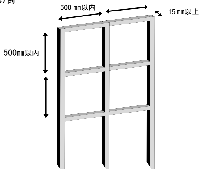
取付け例
